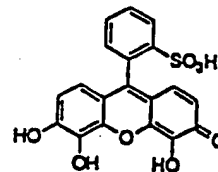
PYROGALLOL RED
